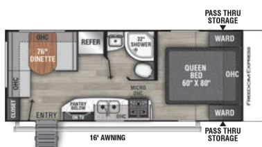
20 SE / Exterior Length 24' 6"
