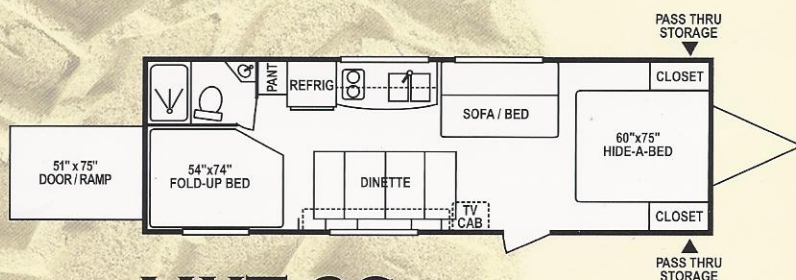
MXT 26
