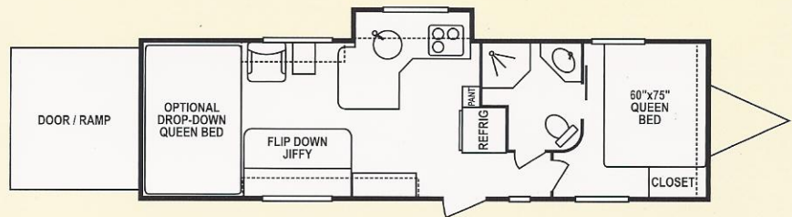
MXT 266
