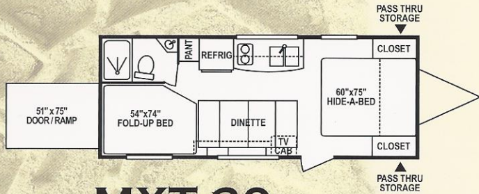
MXT 20
