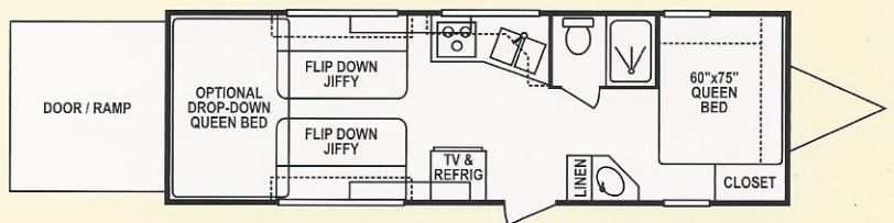
MXT 268
