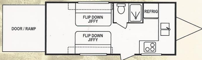
MXT 188
