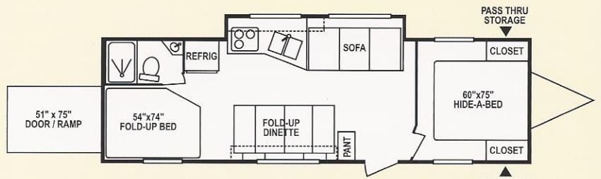
MXT 264R
