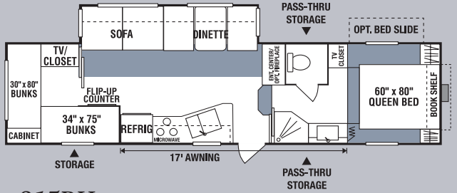
315BH • UVW 8290 • Dry Hitch Wt. 1650 • NCC 1710 • Length 33'5"
