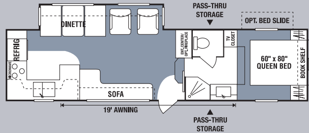
315RK • UVW 8110 • Dry Hitch Wt. 1530 • NCC 1890 • Length 32'5"
