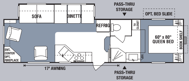
305RE • UVW 7940 • Dry Hitch Wt. 1610 • NCC 2060 • Length 32'11"
