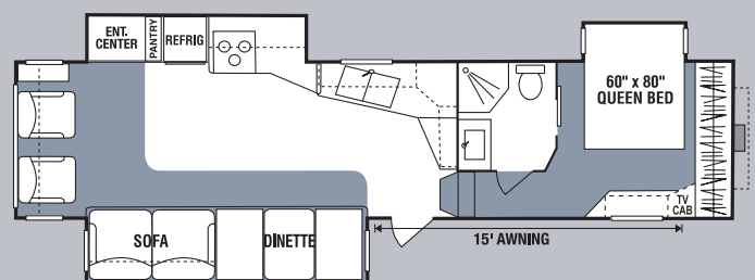
325SB • UVW 9269 • Dry Hitch Wt. 1952 • NCC 1231 • Length 34'10"
