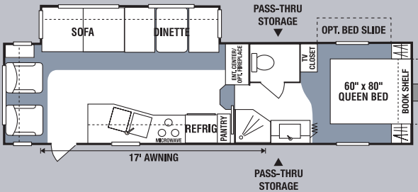
285RL • UVW 7880 • Dry Hitch Wt. 1480 • NCC 1940 • Length 31'1"
