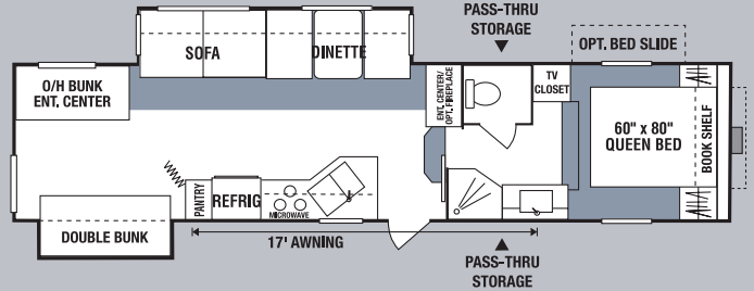
325BH • UVW 8770 • Dry Hitch Wt. 1590 • NCC 1730 • Length 33'5"
