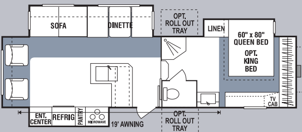
305KS3 • UVW 8796 • Dry Hitch Wt. 2021 • NCC 1204 • Length 32'2"
