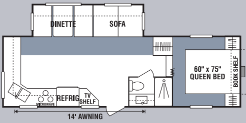
255RK • UVW 6830 • Dry Hitch Wt. 1590 • NCC 2170 • Length 26'3"
