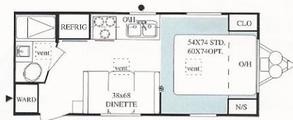
20F - Available Options - 2, 13
