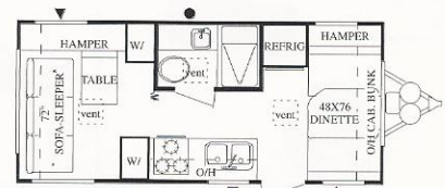
20H - Available Option - 7
