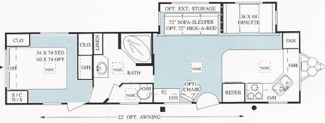
34H Available Option - 6
