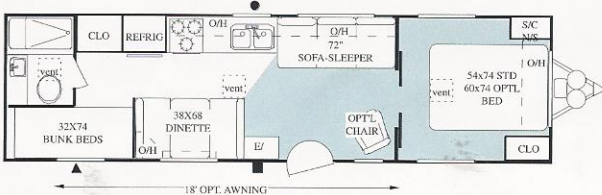
31R Available Option - 2
