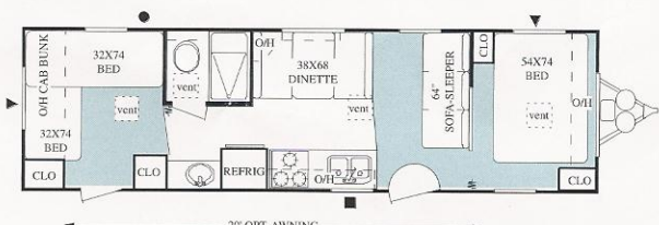
29H Available Options - 7
